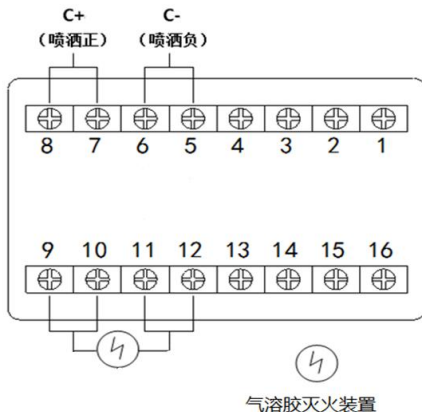
接线示意图
