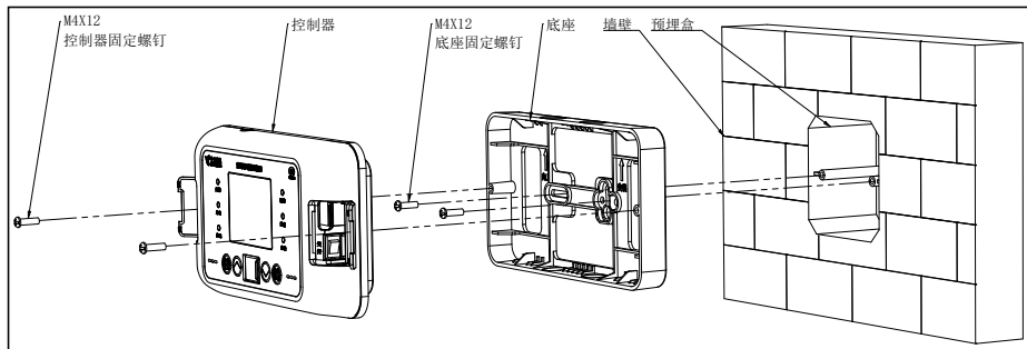
安装示意图
