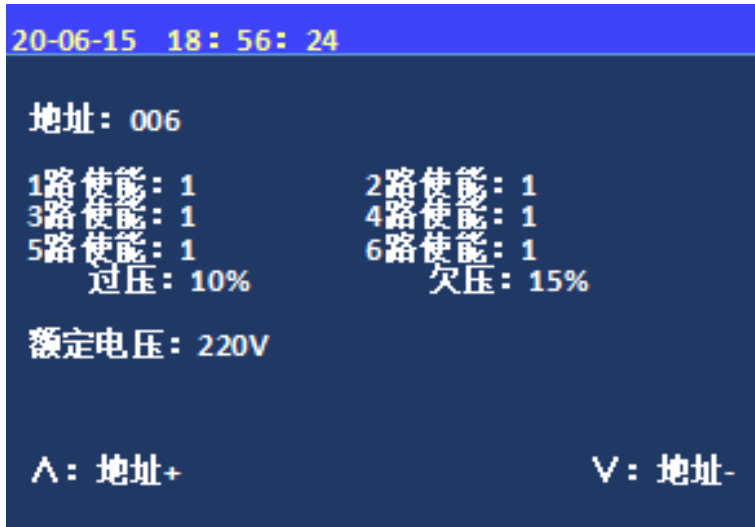
5-1-7 查询传感器参数
