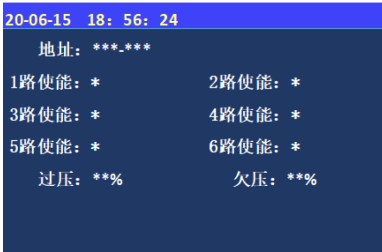
图 5-3-5 设置单相电压参数
