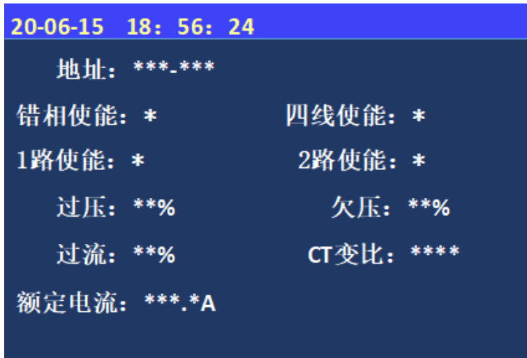
图 5-3-7 设置电压电流参数
