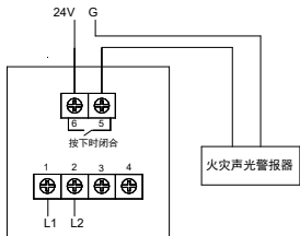
图 2 端子接线图
