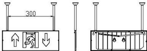
吊装灯具安装示意图
