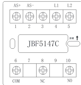
图 2 端子图
